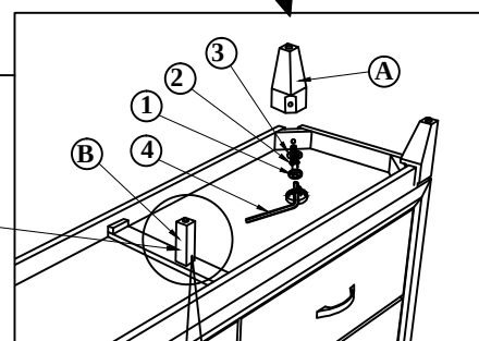
LEVELER ADJUSTER
