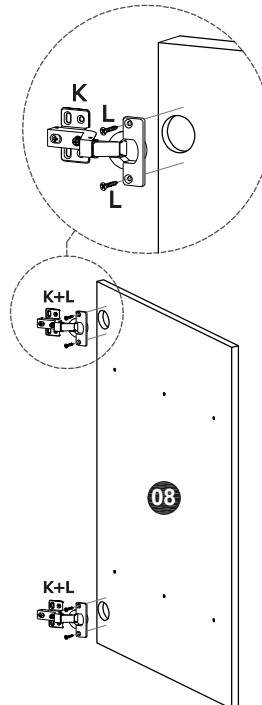
DETAIL 4 / DÉTAIL 4
