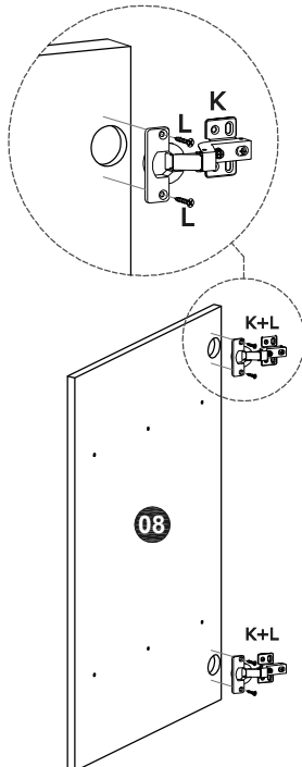
DETAIL 2 / DÉTAIL 2
