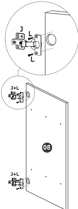
DETAIL 3 / DÉTAIL 3
